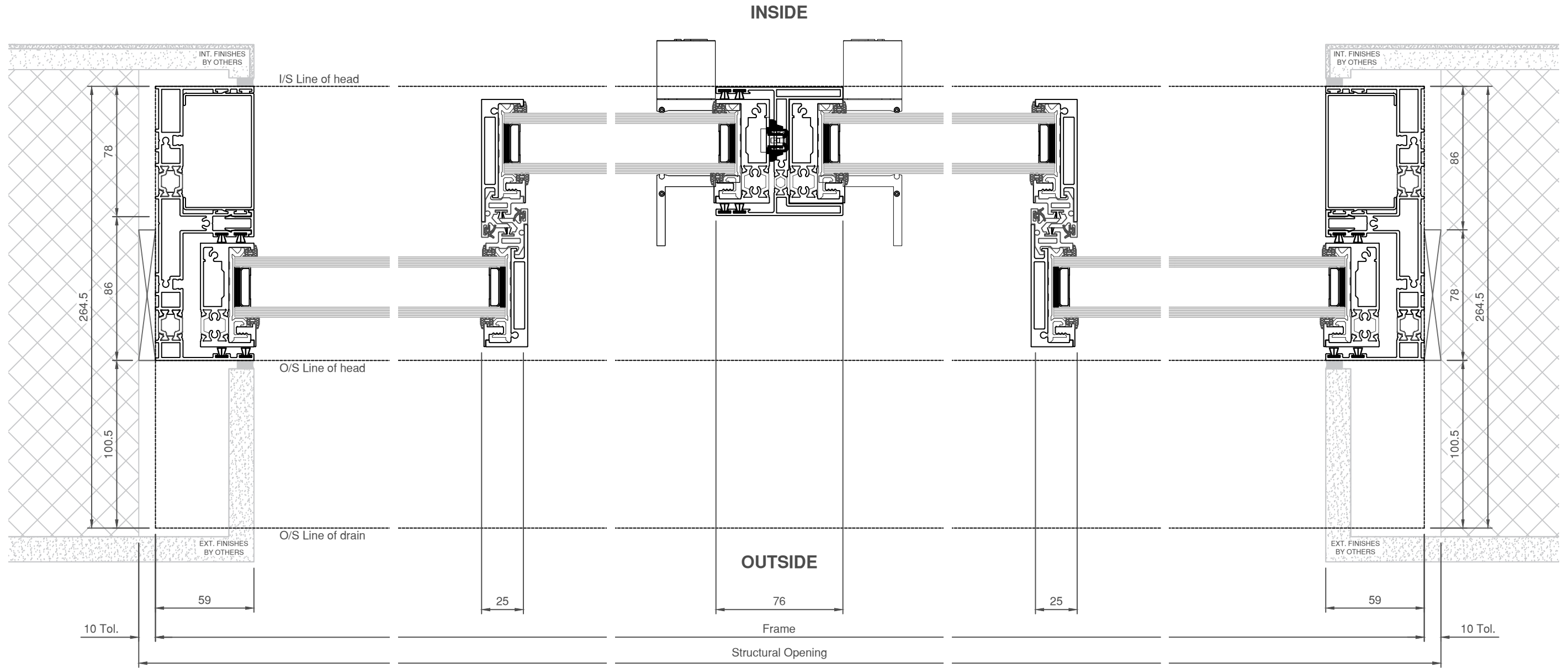
SECTION A-A
